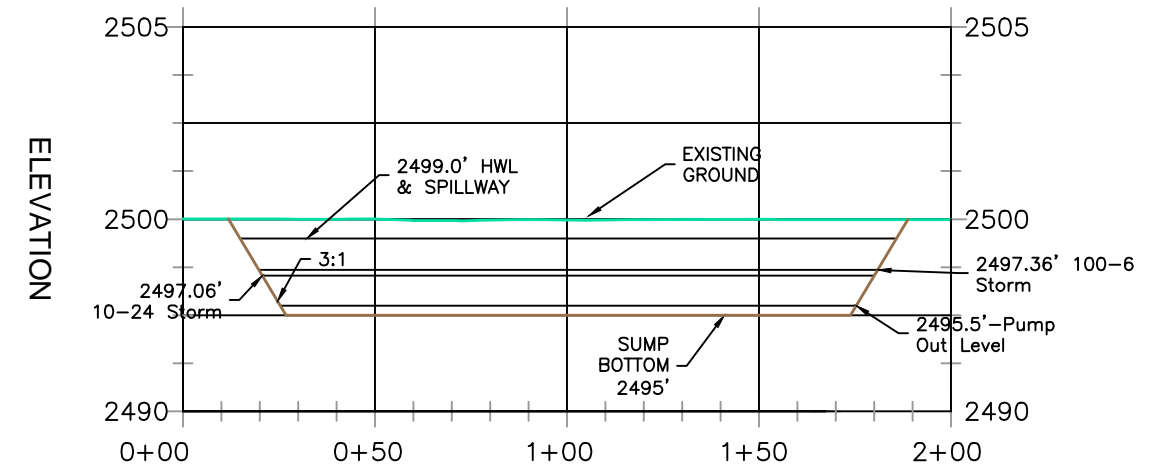
SUMP PROFILE E - E' SCALE: 1"=50'
